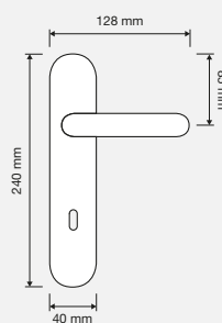
COD. 745 PL
