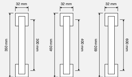
COD. 1555 MN 300 Interassi disponibili / available distances 300 - 400 - 600
